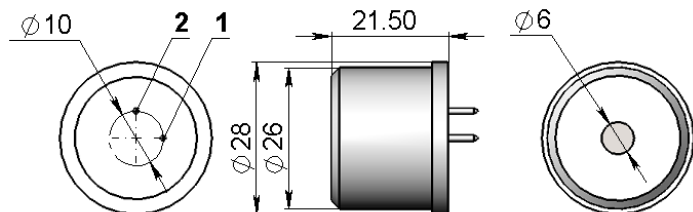
Рис.1 Размеры сенсора и схема расположения выводов 1 - индикаторный электрод 2 - вспомогательный электрод
