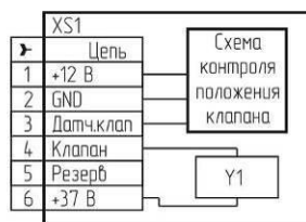
б) с разъемом PГ1Н-1-3
