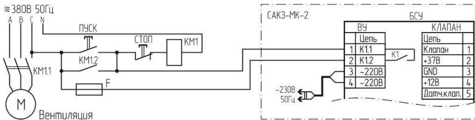
Рисунок Б.3 – Типовая схема соединений для клапанов типа КПЭГ/MADAS EVPS
