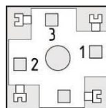
Вилка на кабель PШ2Н-1-17, нумерация контактов (вид со стороны пайки)
