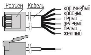
Вилка на кабель TR6P6C Нумерация проводов
