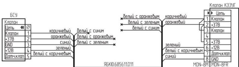
Рисунок Б.7 – Схема подключения клапана КЗЭУГ с разъемом MDN-8FR.
