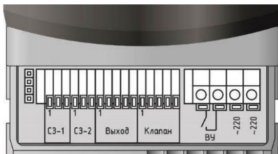
Рисунок 2 – Внешний вид клеммного отсека
