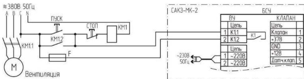
Рисунок А.1 – Типовая схема включения БСУ
